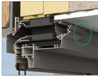
Clapet intérieur divisé Invisivent ®EVO HR
