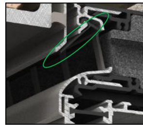
Clapet autoréglable Invisivent EVO AK Basic Invisivent EVO AK High Invisivent EVO AK Ultra
