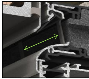
Pas de perforation 80mm Invisivent EVO AK Ultra
